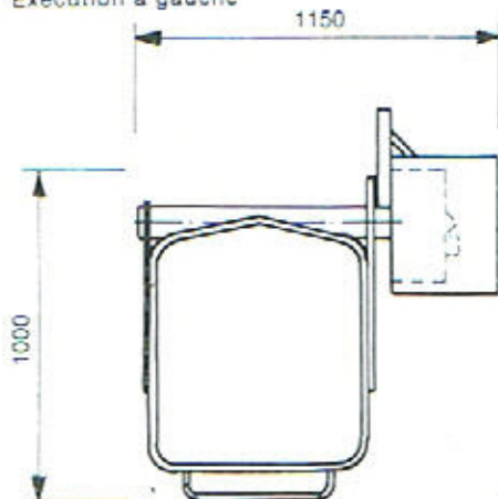
Venstrevendt Left execution Link Ausführung Exécution à gauche
