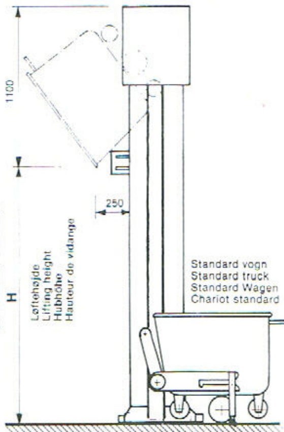
Højrevendt Right execution Recht Ausführung Exécution à droit
